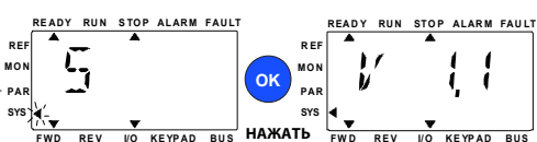
Рис. 19: Главное меню Vacon 20
